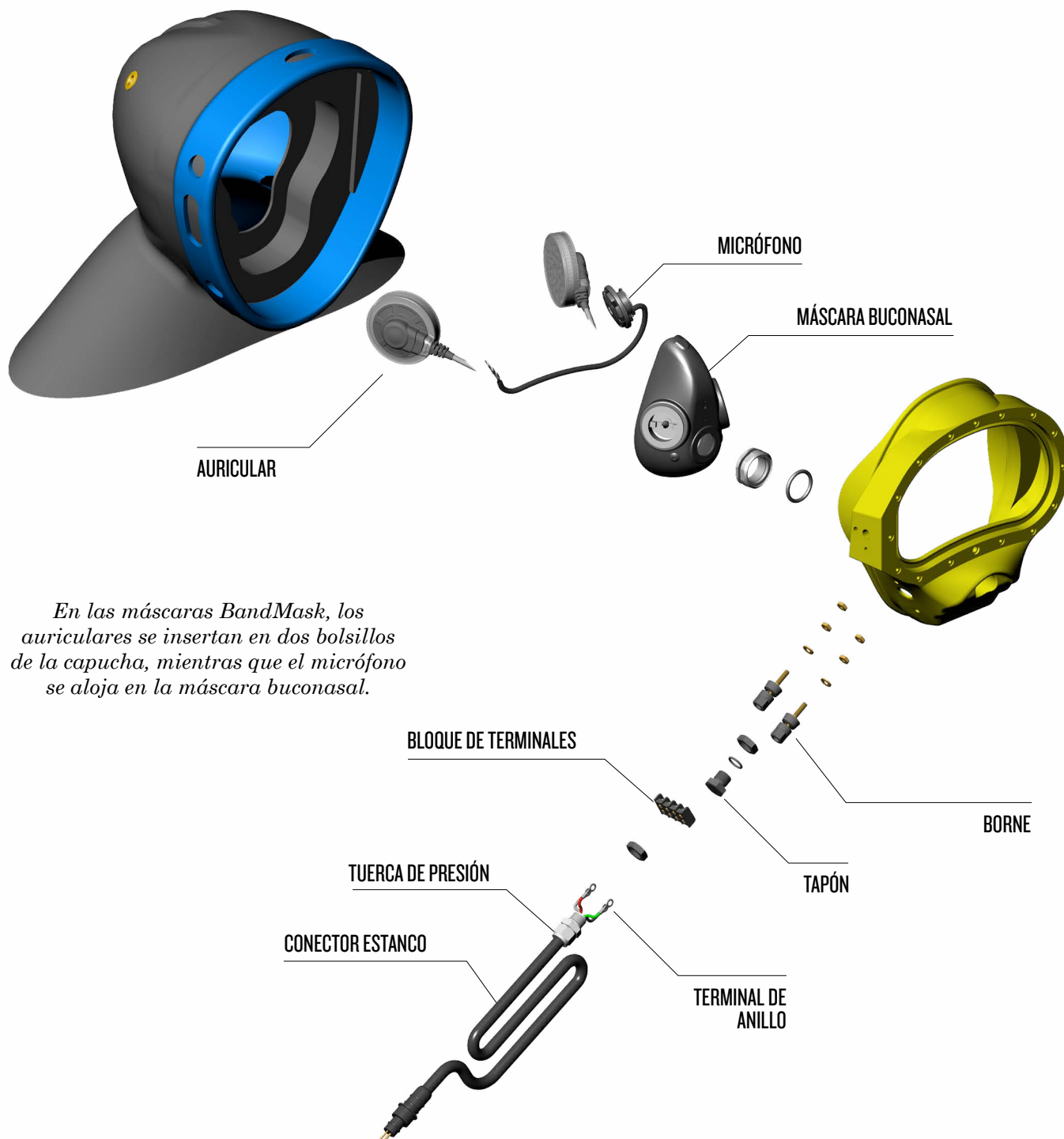
Componentes del conector estanco de los cascos SuperLite® 17B y 17C y las máscaras KMB BandMask
