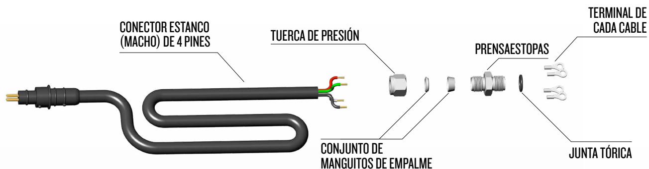
Componentes del conector estanco de los cascos SuperLite® 17B y 17C y las máscaras KMB BandMask
