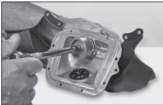
Extracción de la tuerca de montaje del regulador. (Se ha retirado la carcasa para facilitar la observación).
