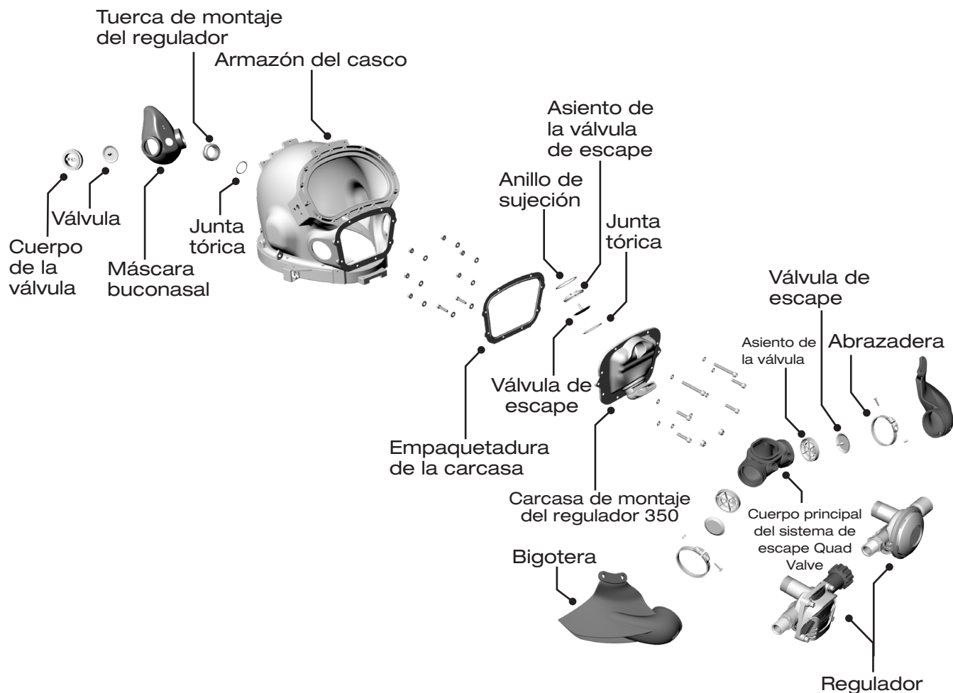
Vista despiezada del regulador SuperFlow® 350 y el regulador compensado 455 con carcasa y máscara buconasal
