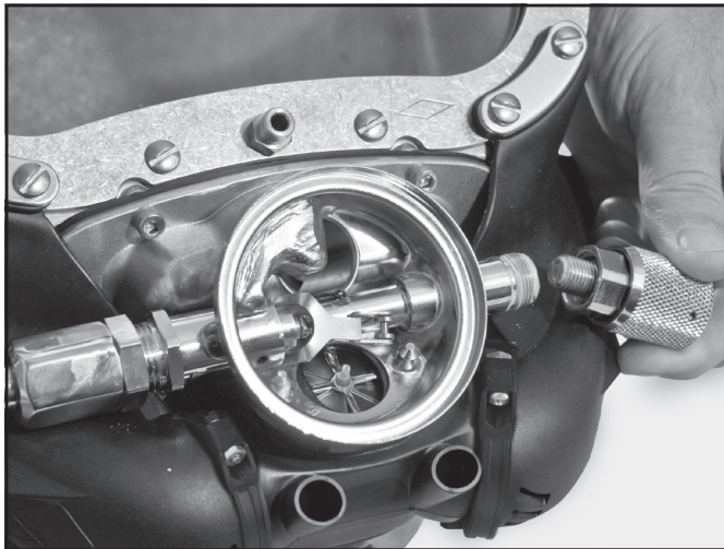
Desenrosque la perilla de ajuste del regulador y quítela.
