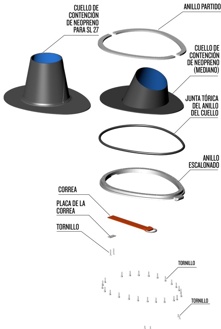
Componentes del anillo del cuello
