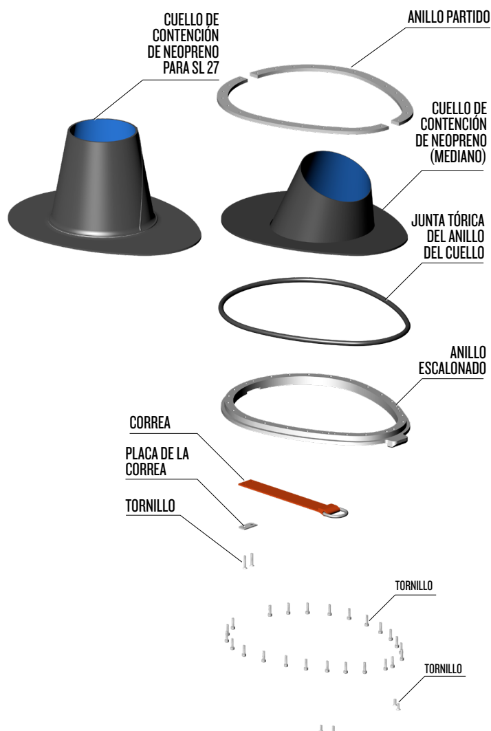
Conjunto de anillos del cuello del casco.
