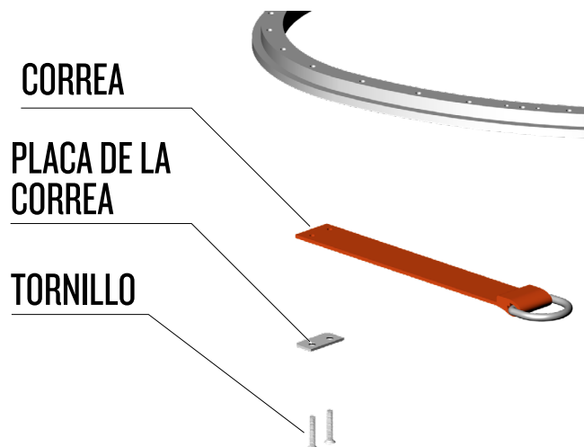
Diagrama de la correa
