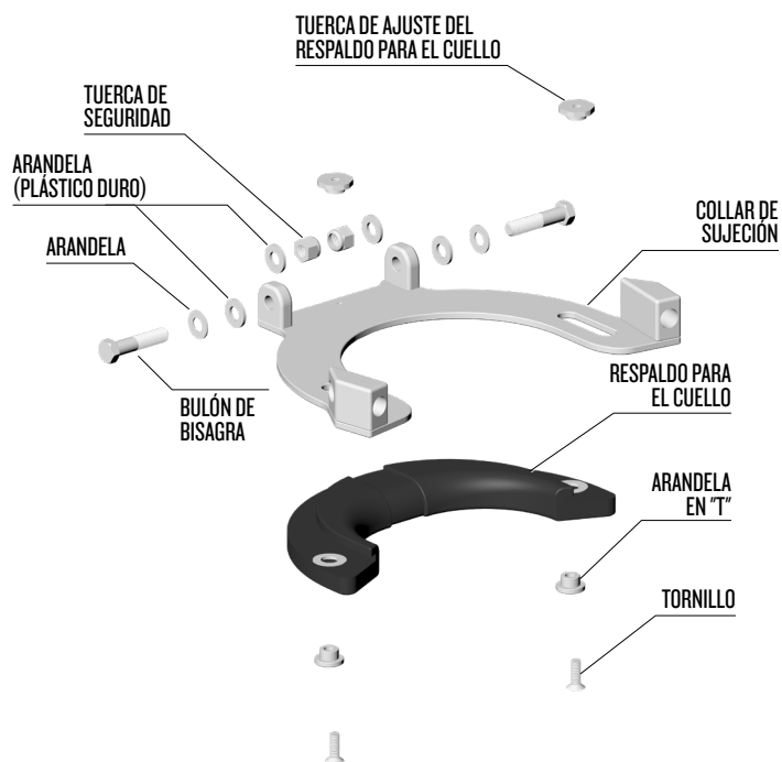
Vista despiezada del conjunto del collar de sujeción
