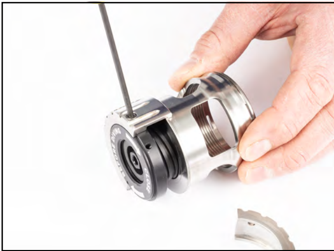
7) Retire la válvula del conjunto del disco.
