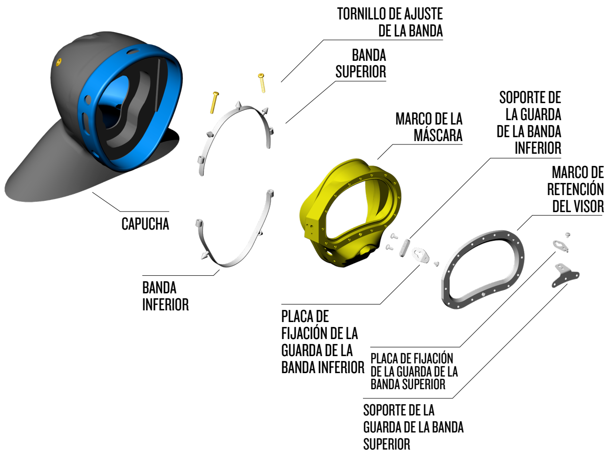
Vista despiezada del sistema de bandas y guardas de las máscaras BandMask
