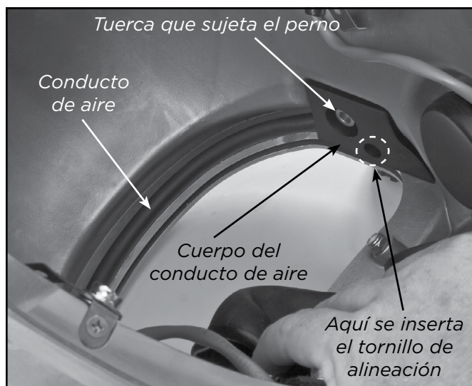
La tuerca de la imagen sujeta tanto el conducto de aire como el bloque lateral.
