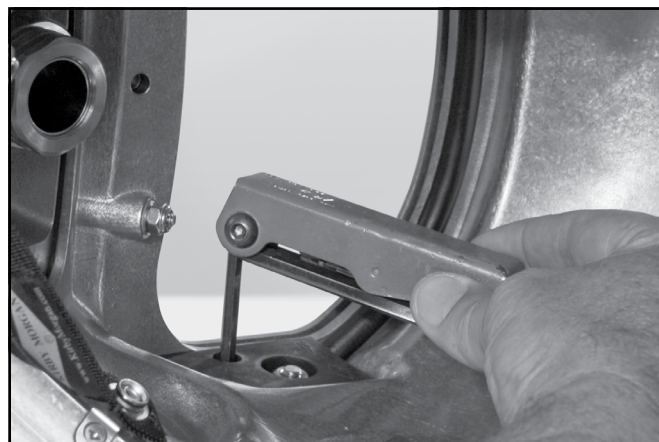
Quite el perno de alineación del interior del cuerpo del conducto de aire.
