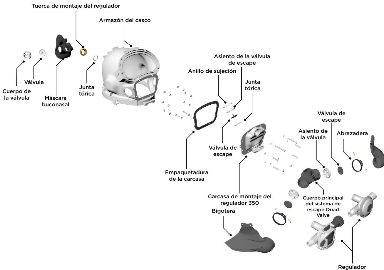
Vista despiezada del regulador SuperFlow® 350 y el regulador compensado 455 con carcasa y máscara buconasal
