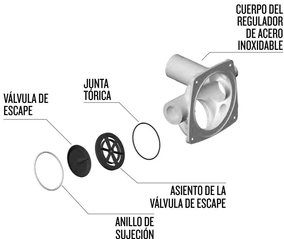
Mecanismo de la válvula de escape del regulador compensado 455
