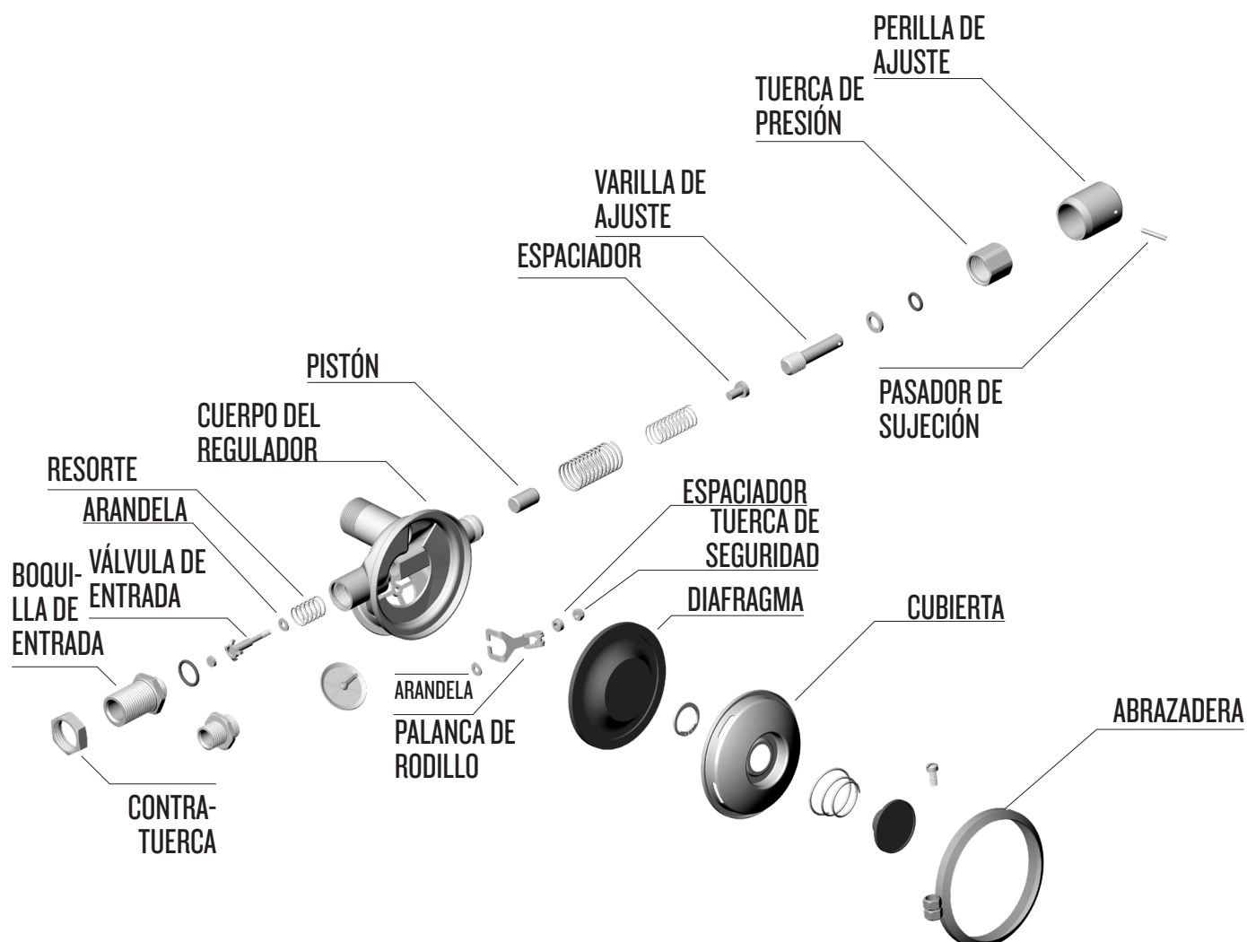
Vista despiezada del conjunto del regulador SuperFlow® (n.º de pieza 505-027)
