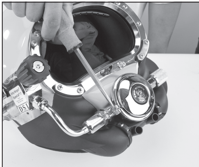
Retire la abrazadera del regulador a demanda.
