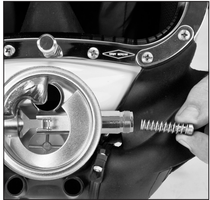
Quite el espaciador, el conjunto de resortes y el pistón.
