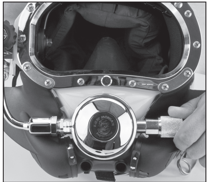
El regulador debería comenzar a producir un flujo libre una vez que se haya girado la perilla de ajuste varias veces hacia afuera.
