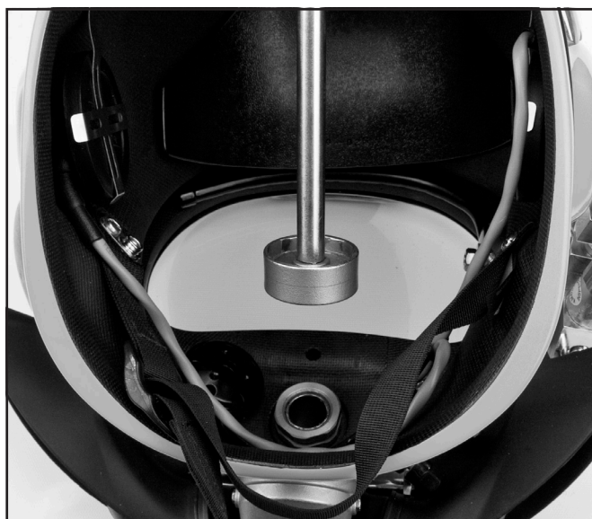
La tuerca de montaje del regulador se debe aflojar con una llave.
