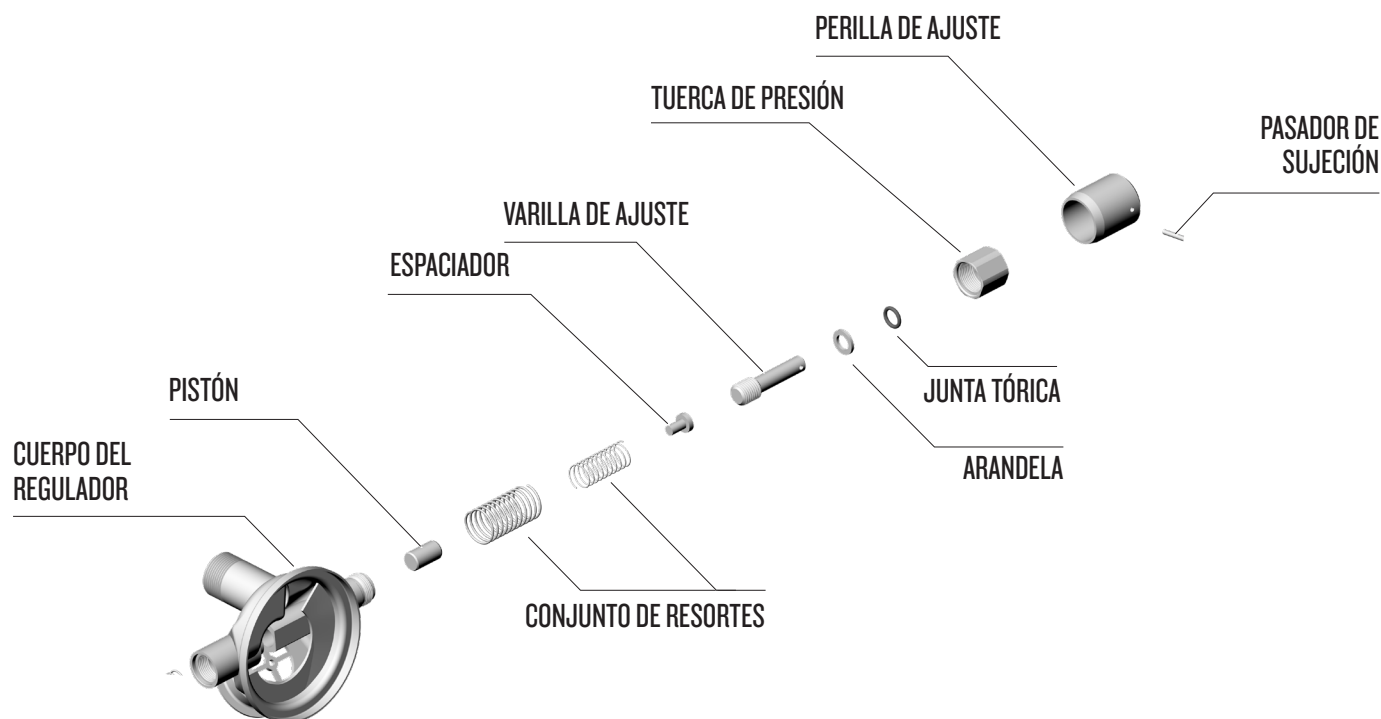
Mecanismo de ajuste del regulador SuperFlow®
