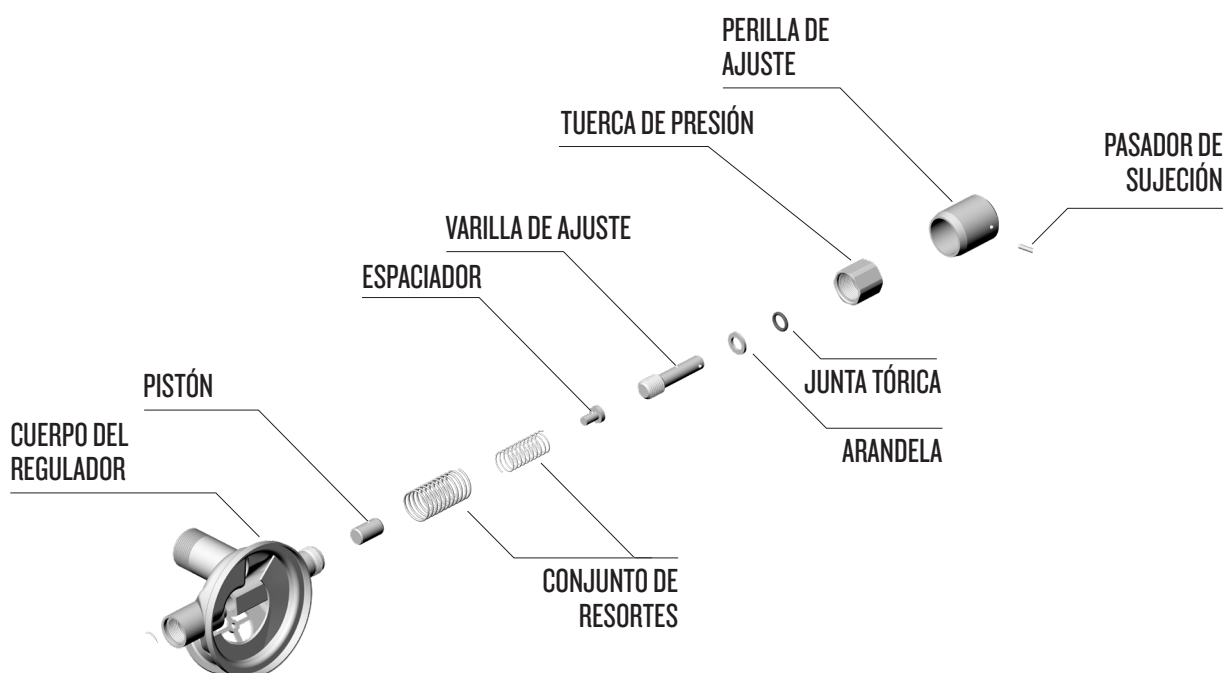
Extremo de ajuste del regulador SuperFlow®
